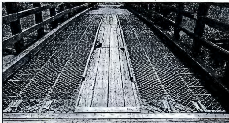
Pokład górny mostu widok ogólny SMT-1
